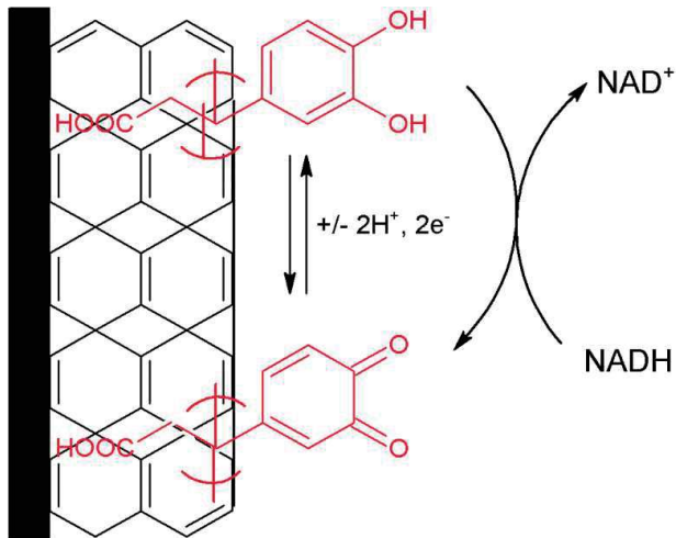
Schemat 1. Katalityczne utlenienie NADH na powierzchni elektrody modyfikowanej MWCNT i katalizatorem zawierającym grupy chinonowe; MWCNT – wielościenna nanorurka węglowa.
