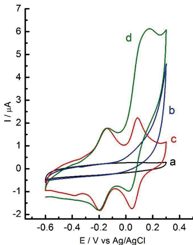
Ryc. 3. Voltamperogramy cykliczne zarejestrowane w buforze fosforanowym (pH = 7,4) dla elektrod GC/SWCNT (a) i GC/SWCNT/PzNO 2 (c) bez dodatku NADH. Krzywe (b) i (d) zarejestrowane zostały na elektrodach GC/SWCNT i GC/SWCNT/PzNO 2 w obecności 1 mM NADH [H3]; GC – elektroda węglowa, SWCNT - jednościenne nanorurka węglowa, PzNO 2 – badana pochodna porfirazyn z grupami nitowymi w podstawnikach peryferyjnych.
