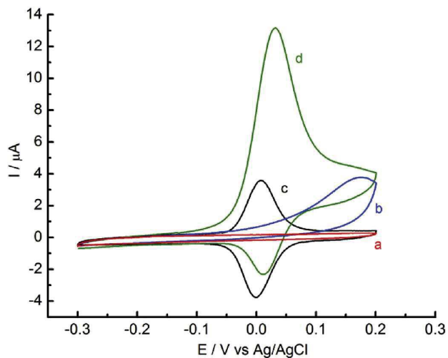
Ryc. 1. Voltamperogramy cykliczne zarejestrowane w buforze fosforanowym (pH 7,4): (a,c) brak NADH i (b,d) w obecności 2 mM NADH dla GC/MWCNT/AAQ/CAT (c, d) i dla GC/MWCNT (a, b) [H 1 ]; GC – elektroda węglowa, MWCNT - wielościenna nanorurka węglowa, AAQ - 1-aminoantrachinon.
