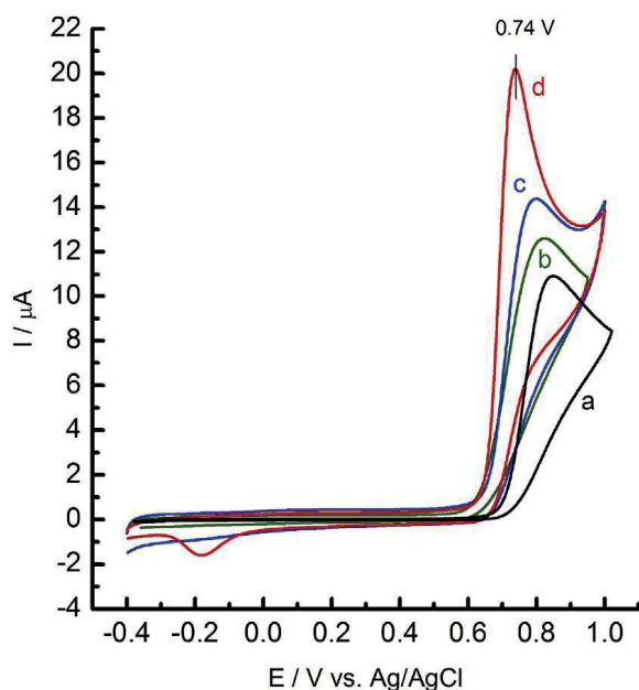
Ryc. 4. Woltamperogramy cykliczne zarejestrowane w buforze fosforanowym (pH = 7,4) dla elektrod GC (a) i GC/Pz (b) GC/SWCNT (c) i GC/SWCNTPz (d) w obecności 1 mM NaNO 2 [H6]; GC – elektroda węglowa, SWCNT - jednościennej nanorurka węglowa, Pz- pochodna porfirazynowa.
