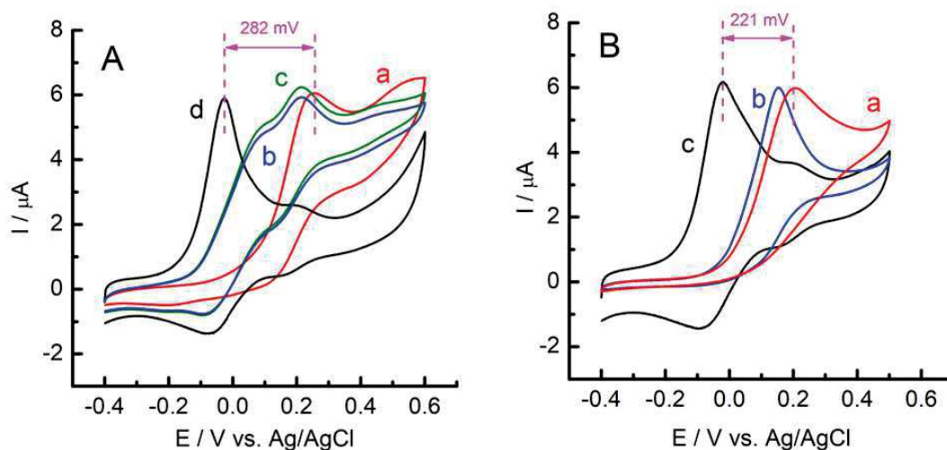
Ryc. 2. (A) Voltamperogramy cykliczne dla GC/PCA 10h @MWCNT, (a), GC/PCA 12h @MWCNT (b), GC/PCA 16h @MWCNT (c) and GC/PCA 24h @MWCNT (d) zarejestrowane w buforze fosforanowym (pH = 7.4) w obecności 2 mM NADH. (B) Voltamperogramy cykliczne dla GC/EPCA@MWCNT (a), GC/CA ads @MWCNT (b) i GC/PCA 24h @MWCNT (c) w obecności 2 mM NADH [H2]; GC – elektroda węglowa, MWCNT - wielościenna nanorurka węglowa, PCA - poli-(kwas kawowy).
