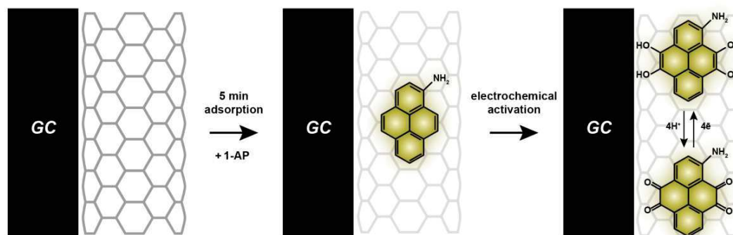
Schemat 4. Elektrochemiczna aktywacja 1-aminopirenu (1-AP) na elektrodzie GC/MWCNT prowadząca do powstania 1-amino-piren-4,5,9,10-tetrolu (1-APox); GC – elektroda węglowa, MWCNT - wielościenna nanorurka węglowa [H4].
