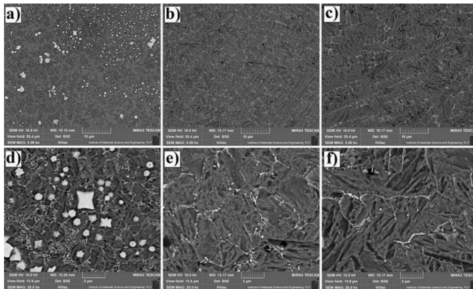
Rys. 35. Mikrostruktura warstw powierzchniowych Fe/TaC - środkowy obszar strefy przetopionej uzyskany przez przetopienie powłoki wstępnej o grubości 90 μm oraz gęstości mocy wiązki lasera: a), d) 64 kW/cm 2 ; b), e) 102 kW/cm 2 oraz c), f) 140 kW/cm 2 – na podstawie [A9]
