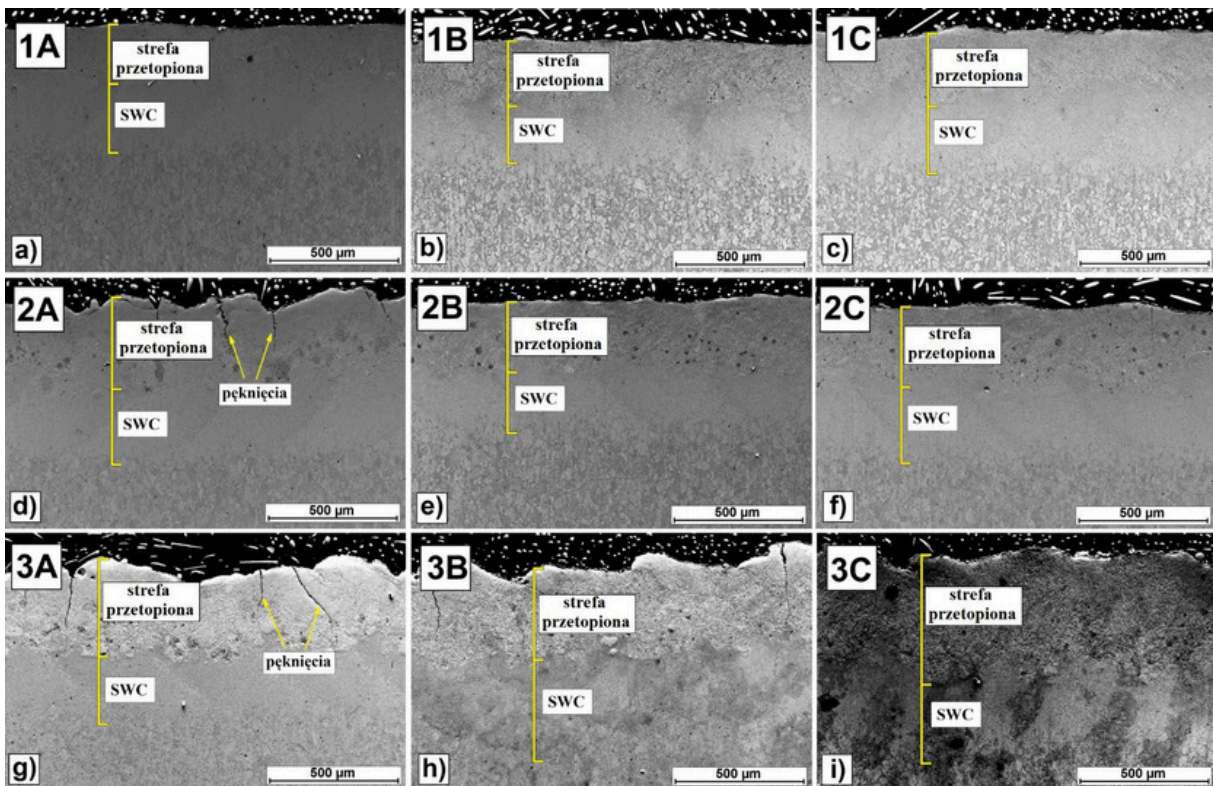
Rys. 28. Morfologia warstw powierzchniowych Fe/ZrC wytwarzanych przy różnych grubościach powłoki wstępnej: 1 - 100 \mu\text{m} , 2 - 150 \mu\text{m} , 3 - 200 \mu\text{m} oraz przy różnych gęstościach mocy wiązki lasera: A - 64 \text{kW}/\text{cm}^2 , B - 89 \text{kW}/\text{cm}^2 , C - 115 \text{kW}/\text{cm}^2 – na podstawie [A7]
