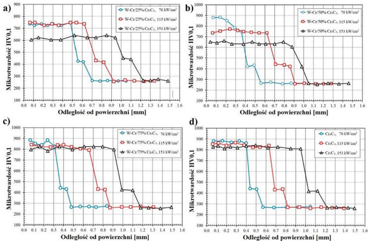
Rys. 11. Profile mikrotwardości dla warstw wytwarzanych przy trzech gęstościach mocy wiązki lasera 76 kW/cm 2 , 115 kW/cm 2 oraz 153 kW/cm 2 oraz przy różnych stężeniach fazy wzmacniającej: a) 25% Cr 3 C 2 , b) 50% Cr 3 C 2 , c) 75% Cr 3 C 2 oraz d) 100% Cr 3 C 2 – na podstawie [A3]
