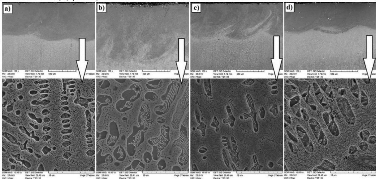
Rys. 15. Warstwy powierzchniowe Fe-B/( \text{B}_4\text{C}+\text{Si} ) wraz z ich mikrostrukturą wytworzone przy parametrach: a) 600 mm/min i 30 \text{kW}/\text{cm}^2 , b) 600 mm/min i 40 \text{kW}/\text{cm}^2 , c) 800 mm/min i 30 \text{kW}/\text{cm}^2 , d) 1000 mm/min i 30 \text{kW}/\text{cm}^2 – na podstawie [A4]
