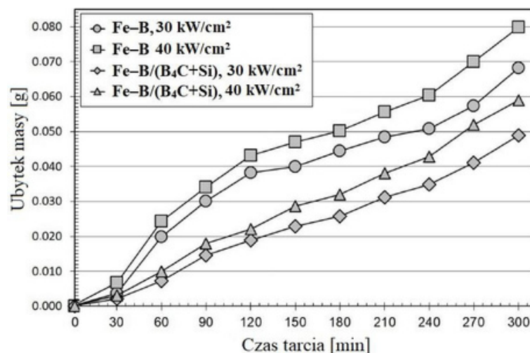
Rys. 17. Odporność na zużycie przez tarcie dla warstw powierzchniowych Fe–B oraz Fe–B/(B 4 C+Si) wytwarzanych przy prędkości skanowania 600 mm/min oraz różnych parametrach gęstości mocy wiązki lasera – na podstawie [A4]
