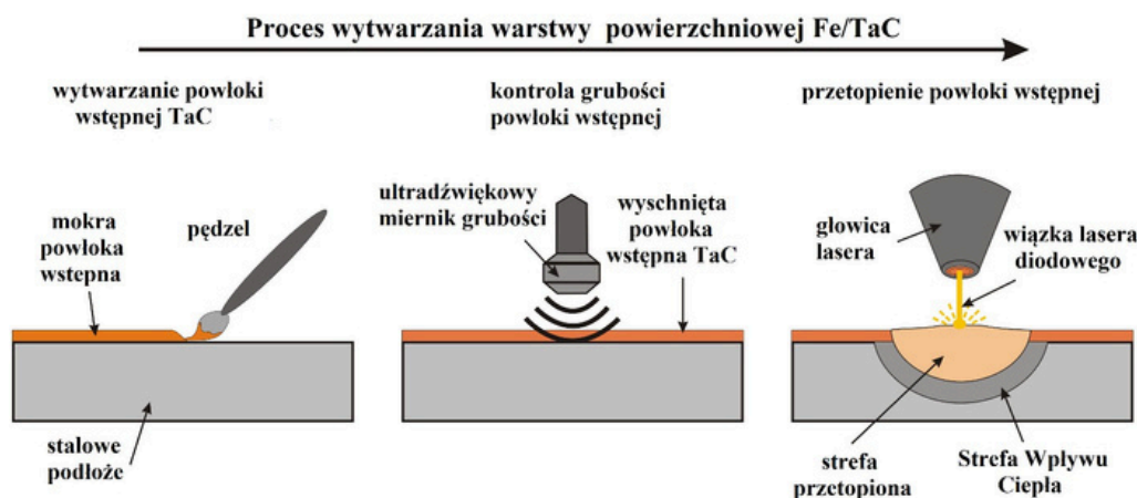
Rys. 34. Schemat wytwarzania warstw Fe/TaC – na podstawie [A9]
