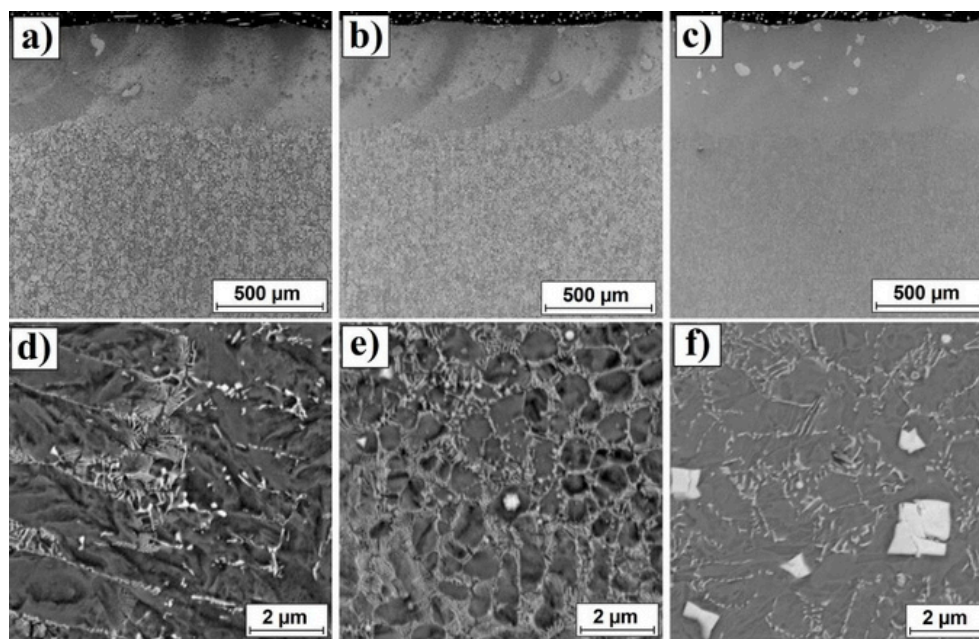
Rys. 38. Mikrostruktura warstw Fe/TaC wytworzonych przy użyciu gęstości mocy 64 kW/cm 2 oraz grubości powłoki wstępnej: a), d) 30 μm; b), e) 60 μm; c), f) 90 μm – na podstawie [A10]
