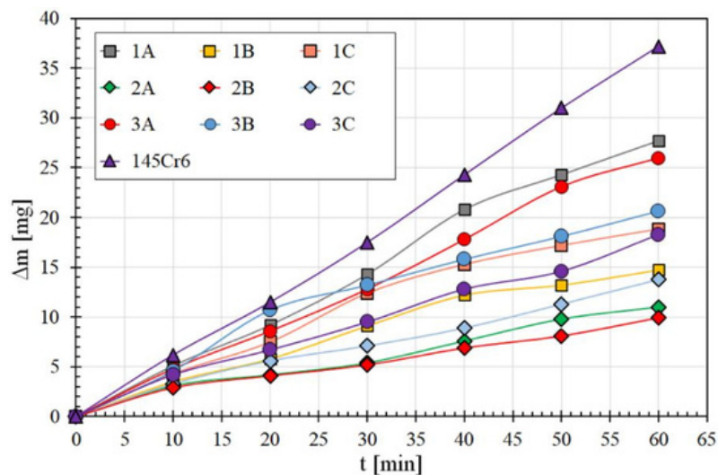
Rys. 30. Odporność na zużycie przez tarcie warstw powierzchniowych Fe/ZrC wytwarzanych przy różnych grubościach powłoki wstępnej: 1 - 100 μm, 2 - 150 μm, 3 - 200 μm oraz przy różnych gęstościach mocy wiązki lasera: A - 64 kW/cm 2 , B - 89 kW/cm 2 , C - 115 kW/cm 2 – na podstawie [A7]
