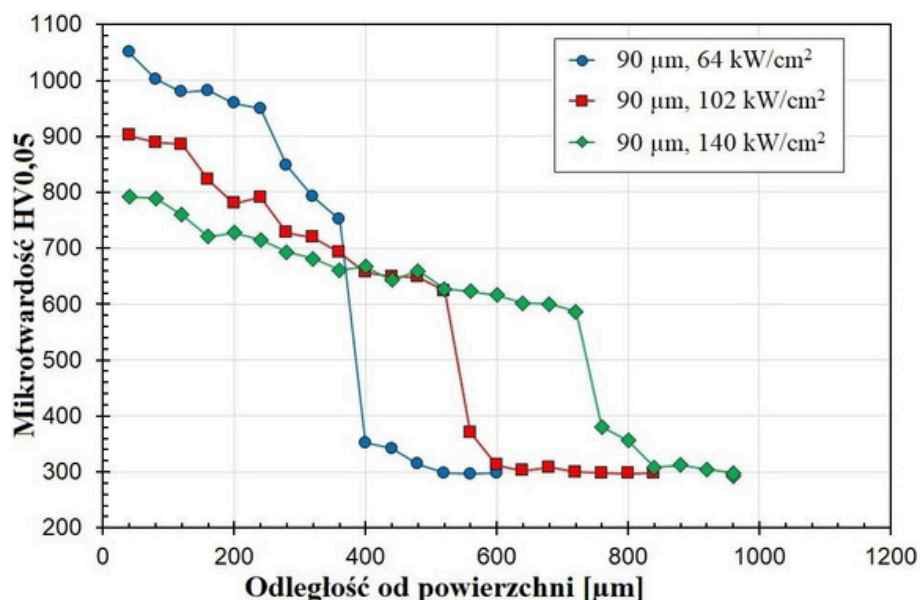
Rys. 37. Mikrotwardość warstw powierzchniowych Fe/TaC uzyskanych przez przetopienie powłoki wstępnej o grubości 90 μm oraz gęstości mocy wiązki lasera: 64 kW/cm 2 , 102 kW/cm 2 oraz 140 kW/cm 2 – na podstawie [A9]
