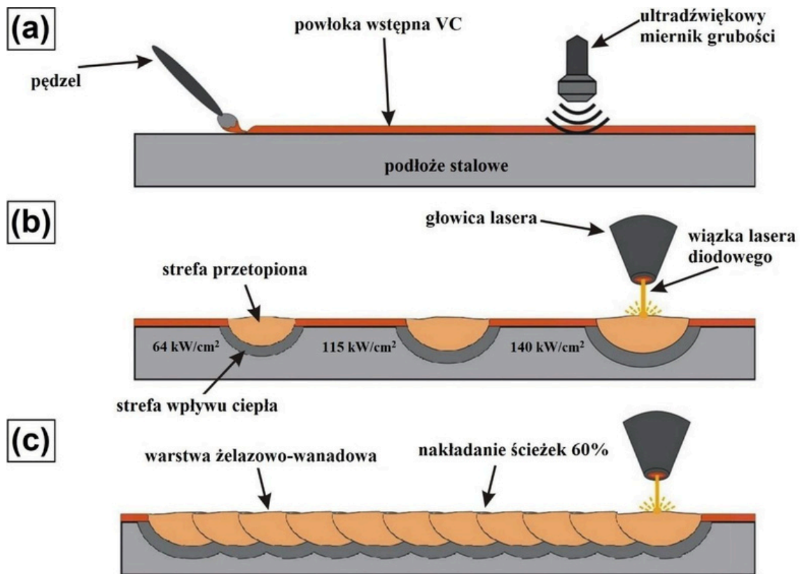
Rys. 40. Schemat wytwarzania warstw powierzchniowych wzmacnianych węglikiem wanadu: a) nakładanie powłoki wstępnej, b) wytwarzanie ścieżek pojedynczych, c) wytwarzanie ścieżek wielokrotnych – na podstawie [A11]
