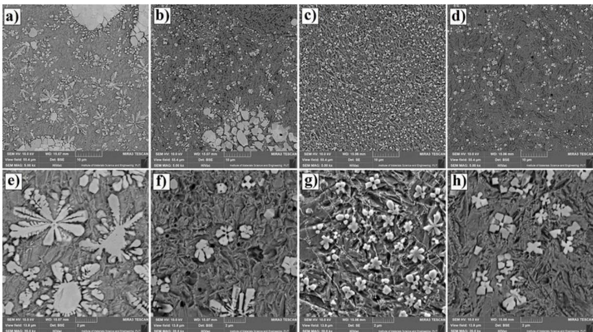
Rys. 25. Środkowy obszar strefy przetopionej w dwóch powiększeniach dla warstw powierzchniowych Fe/ZrC wytworzonych przy gęstości mocy wiązki lasera: a), e) 64 kW/cm 2 ; b), f) 89 kW/cm 2 ; c), g) 115 kW/cm 2 ; d), h) 140 kW/cm 2 – na podstawie [A6]
