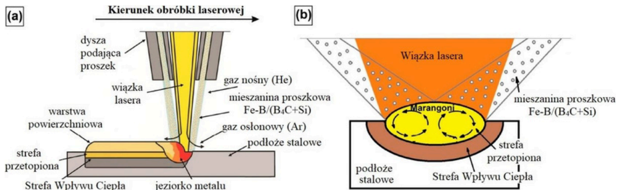
Rys. 13. Wytwarzanie warstw powierzchniowych Fe-B/(B 4 C+Si) metodą proszkowego napawania laserowego: a) schemat metody, b) przedstawienie ruchów konwekcyjnych Marangoni powodujących mieszanie jeziora ciekłego metalu – na podstawie [A4]
