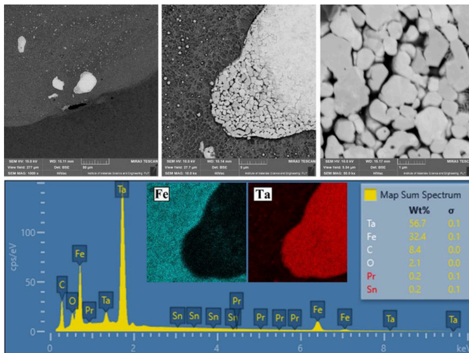
Rys. 36. Aglomeraty powstające w warstwach powierzchniowych Fe/TaC: a) morfologia warstwy, b) powiększenie granicy aglomerat - osnowa, c) powiększenie struktury aglomeratu, d) skład chemiczny aglomeratu – na podstawie [A9]
